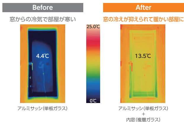
サーモグラフィで見る冬の窓の温度
